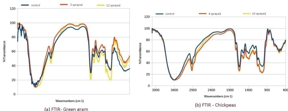
Fig 3: FTIR spectra
