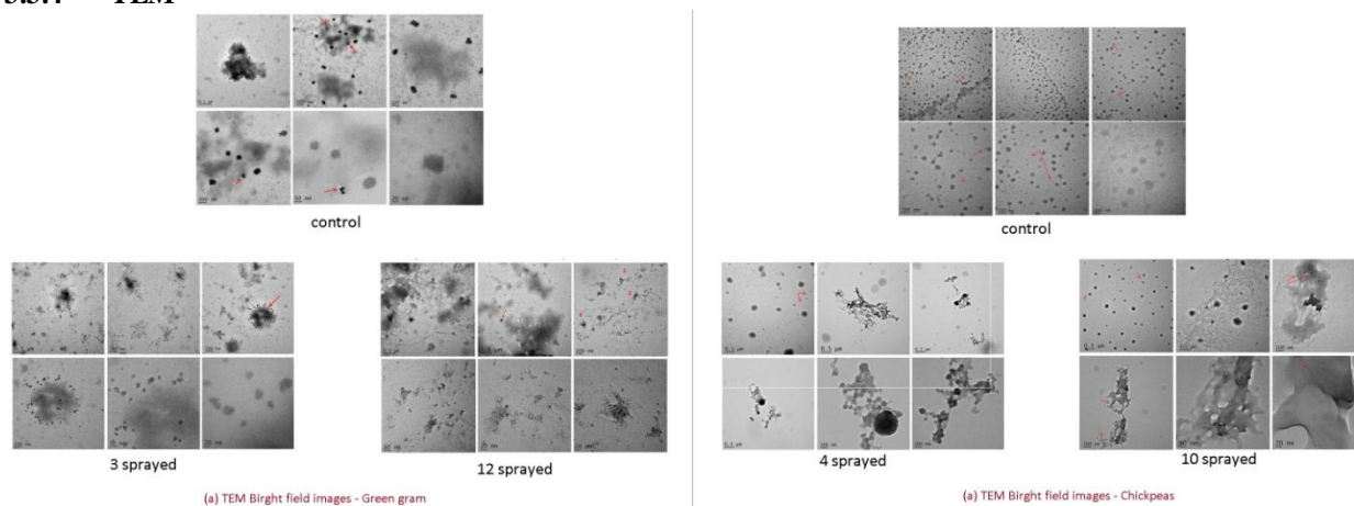
Fig 5: TEM images
