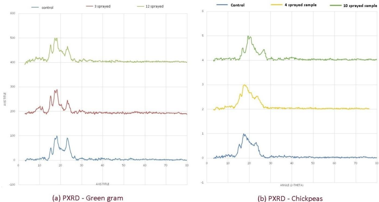
Fig 4: PXRD spectra
